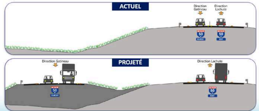
Schéma projeté de la construction d'une 2 e chaussée d'autoroute au nord de la chaussée actuelle. Crédit : Ministère des Transports et de la Mobilité durable.
